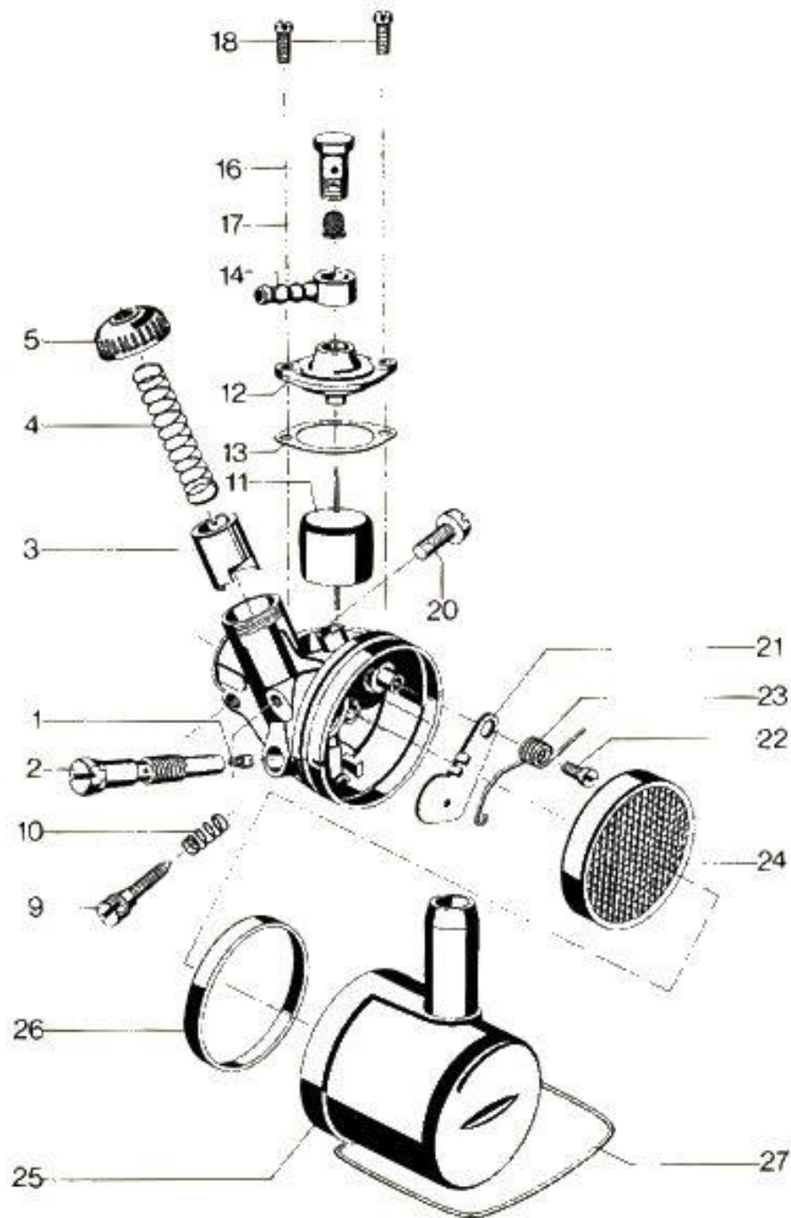
ENCARWI Vergaser S8A, S23, S22, S25, 88S25/101 auf Laura M48 Motor
